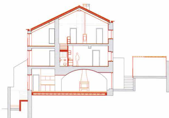
Sezione trasversale
