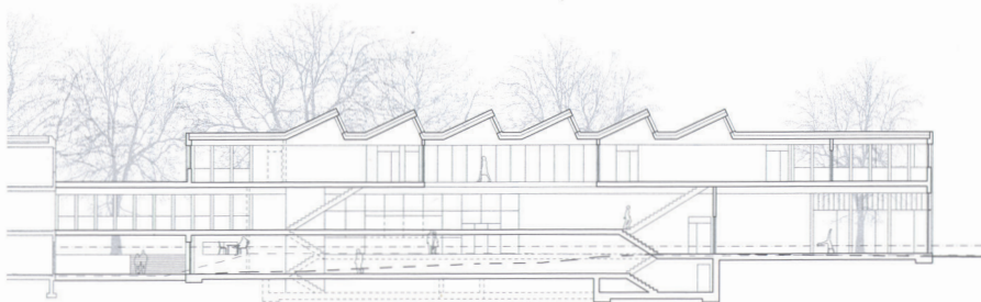
Schnitt, 1:600
