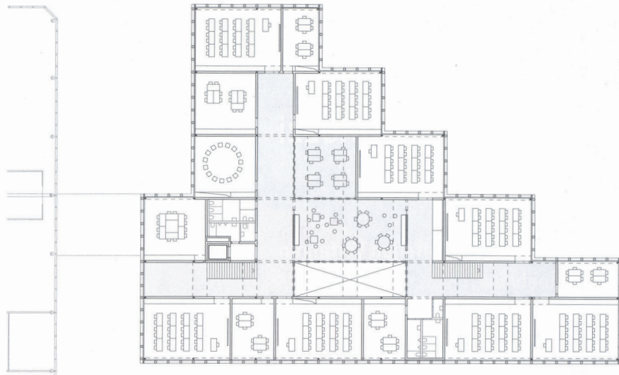
Obergeschoss, 1:600
